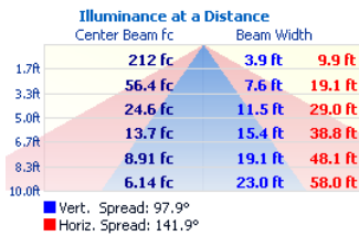
SS-2-L18-SF
