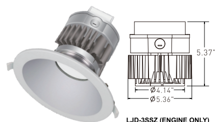
LJD-3SSZ (ENGINE ONLY)
