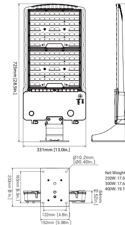
(Wall Mount)
