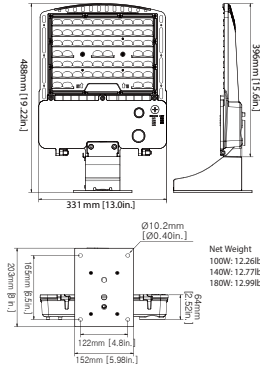
(Wall Mount)
