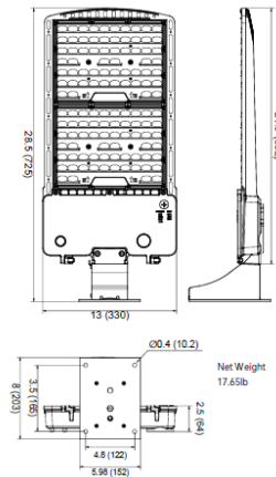
(Wall Mount)
