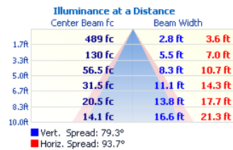
CUBE4-3-D48L-WW
