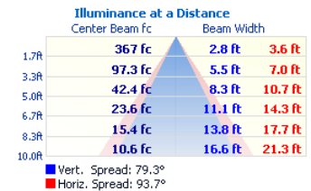
CUBE4-3-D36L-WW
