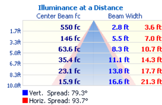
CUBE4-3-D54L-WW
