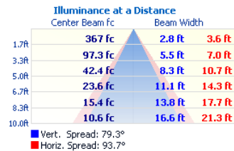
CUBE4-2-D54L-WW
