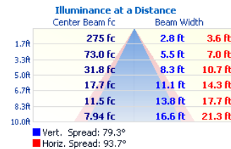
CUBE4-3-D27L-WW
