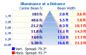
CUBE4-3-D18L-WW
