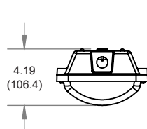
DW-LP
