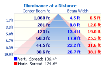
DW-LP-4-72LED
