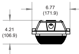
DW-LP
